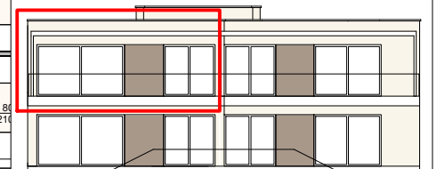
SÜDANSICHT
